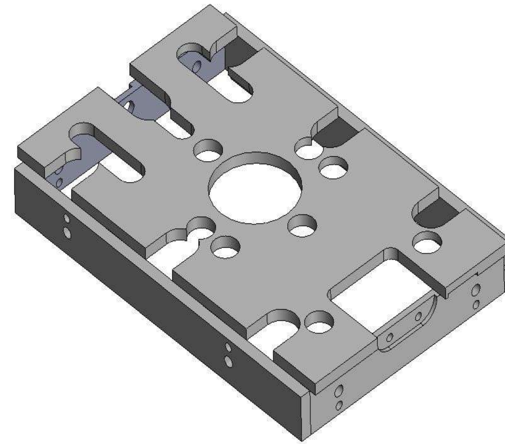
Insulating plate UMAR-P379186 UMAR-P379187 UMAR-P379188 UMAR-P379189 UMAR-P379190 Improved
